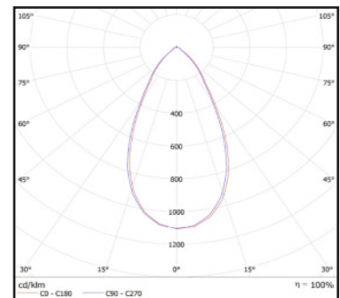
Ljusfördelning 60°
