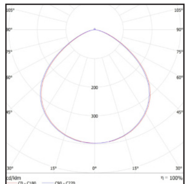
Ljusfördelning 90°
