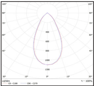
Ljufördelning 60°
