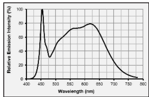
Ljusspektrum 4.000K
