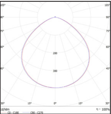
Ljufördelning 90°
