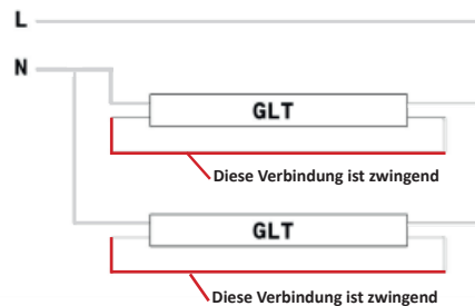
Bild 2: Elektroschema mehrflammig
