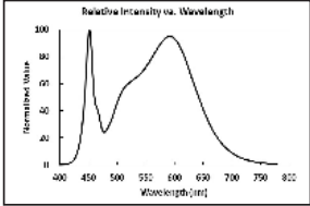
Lichtspektrum 5.000K
