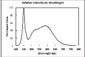
Lichtspektrum 5.000K
