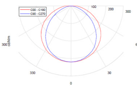
Lichtverteilung
